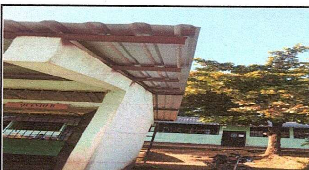
Foto 4: Costaneras reforzadas y pintadas.
